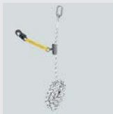
Mitlaufendes Auffanggerät am Führungsseil
