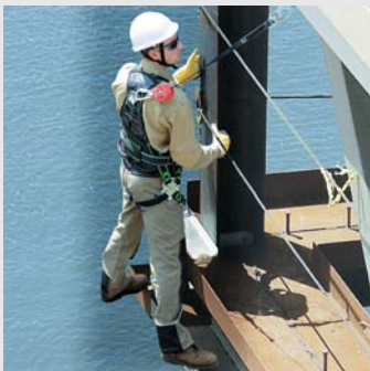
Mitlaufendes Auffanggerät am Führungsseil
