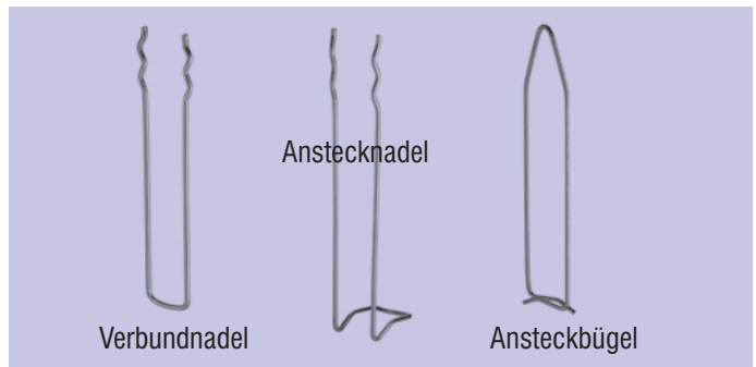
Verbundankernadeln
