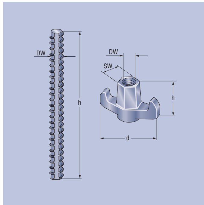
Abbildung der Flügelmutter typähnlich
